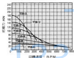
把握力性能曲線 TF3B
